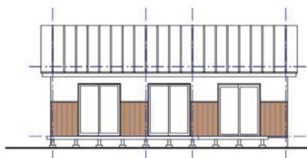
南立面図
