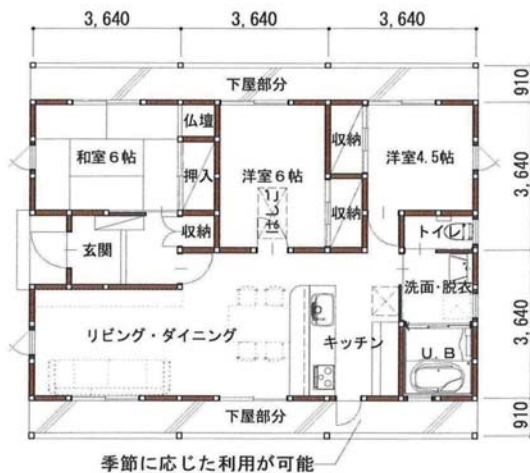
1 階平面図
